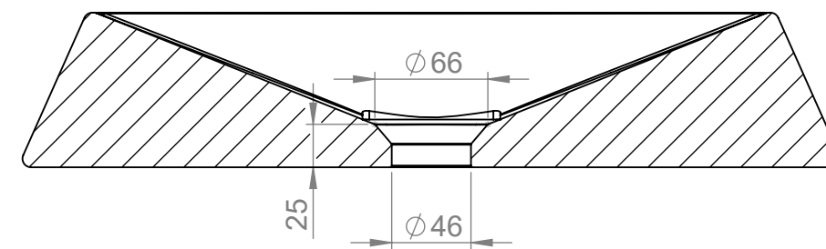
PRZEKRÓJ A-A
