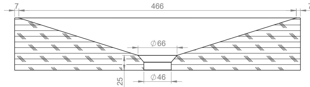
PRZEKRÓJ A-A
