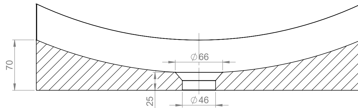
PRZĘKRÓJ A-A
