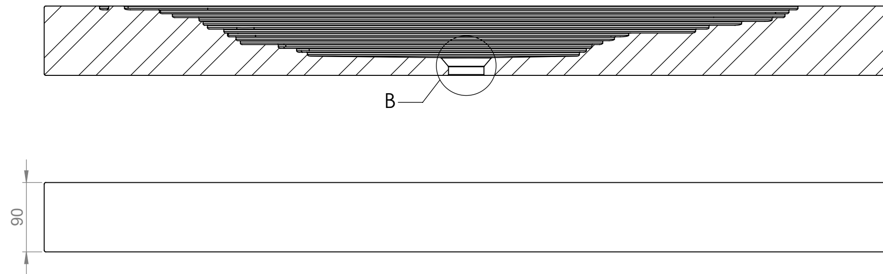
PRZEKRÓJ A-A
