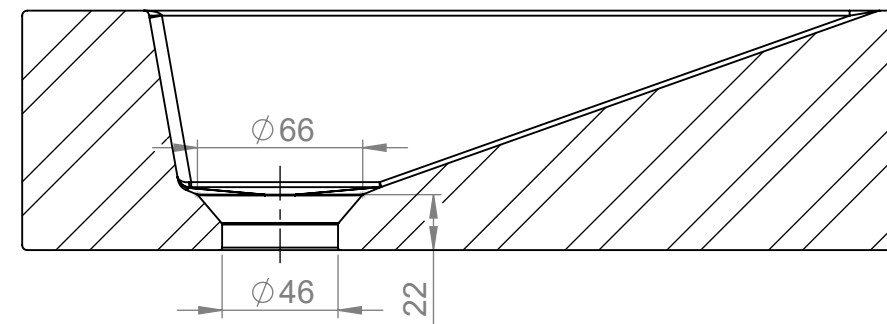
PRZEKRÓJ A-A
