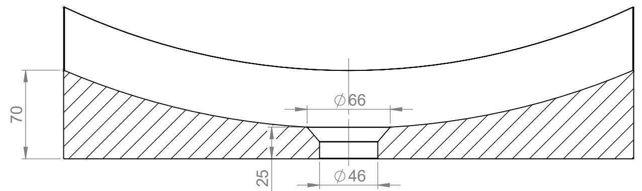
PRZEKRÓJ A-A
