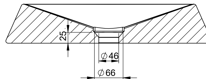
PRZĘKRÓJ A-A
